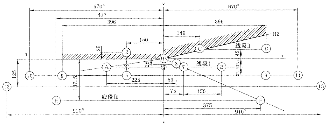
测量屏幕 I 近光
