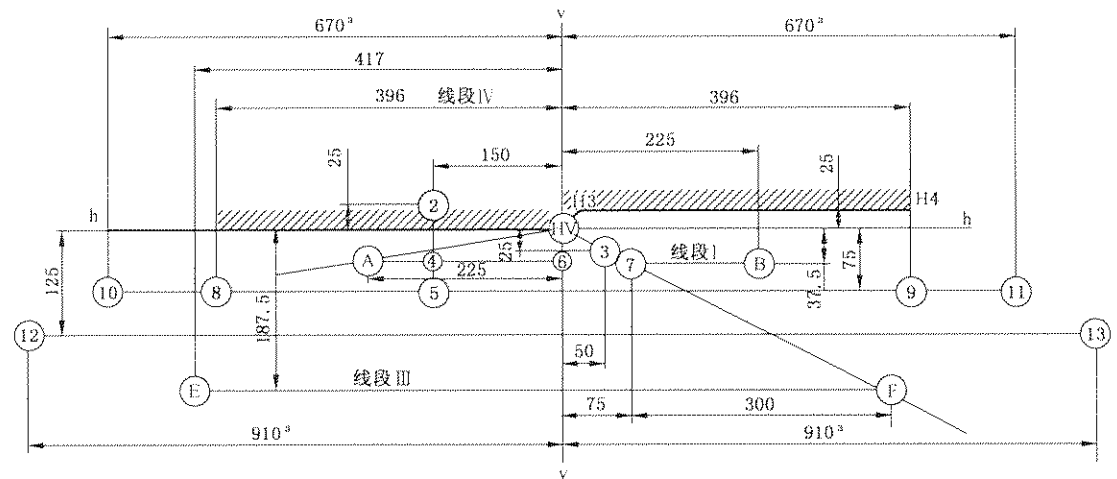
测量屏幕 II 近光
